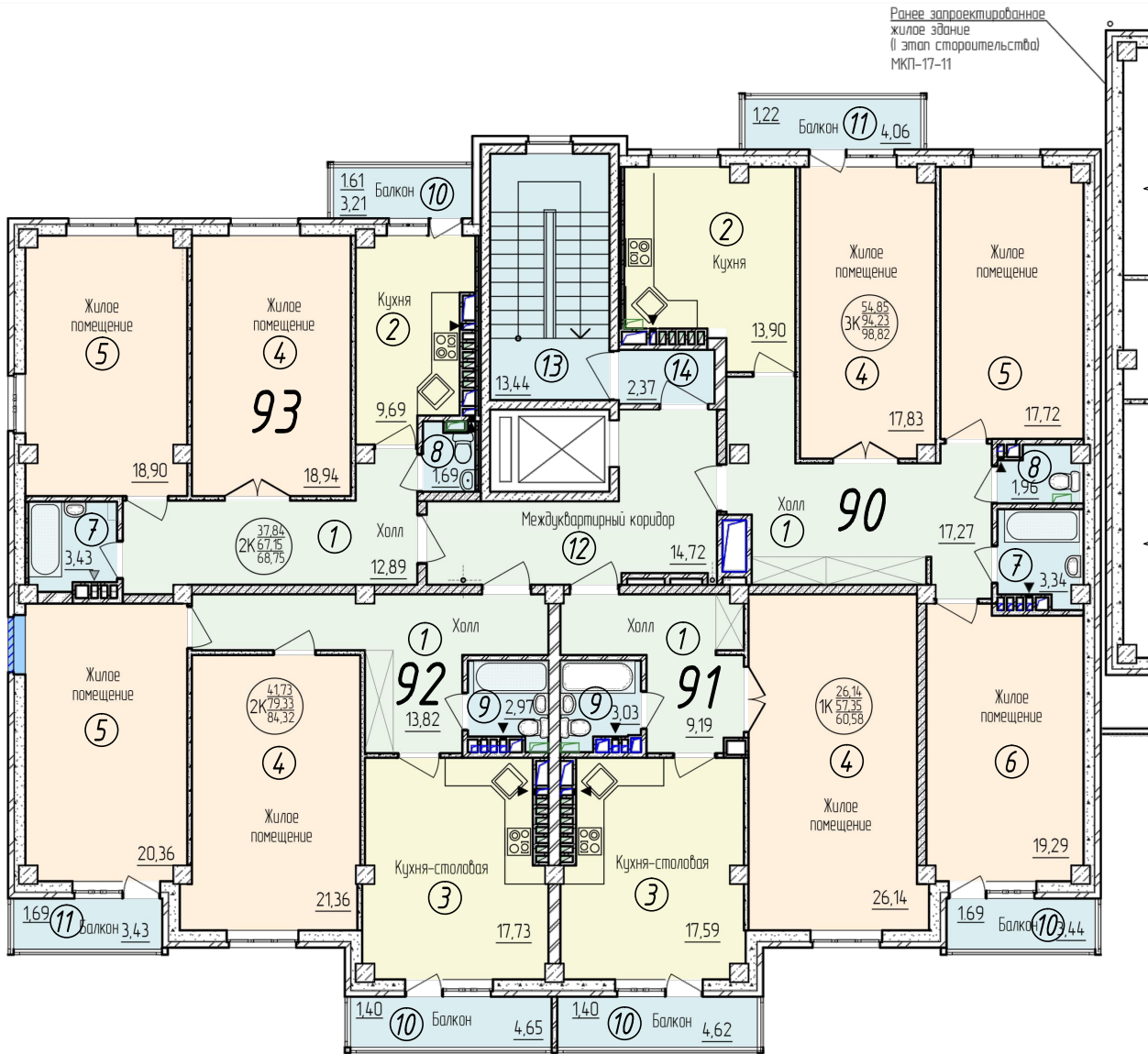
План 4 этажа
